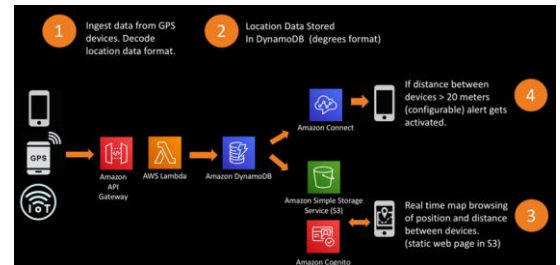
그림(5) Entire Block Diagram
