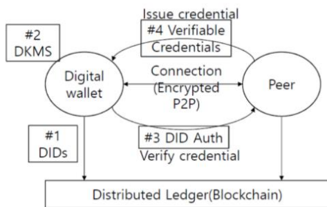
(그림 4) DID 기술 구성도
