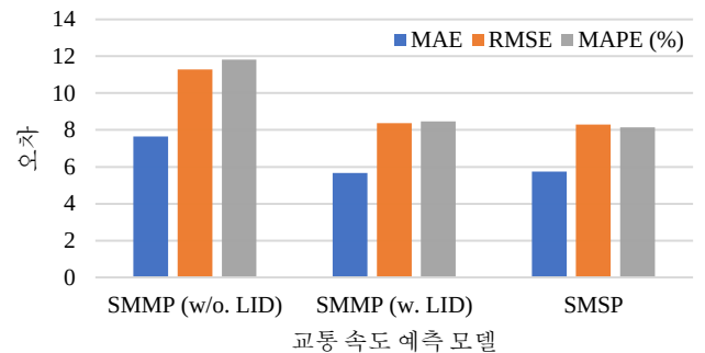
(그림 2) LID 사용 여부에 따른 SMMP 및 SMSP의 정확도.
