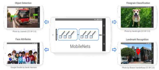
그림 3. MobileNet 구조[5].
