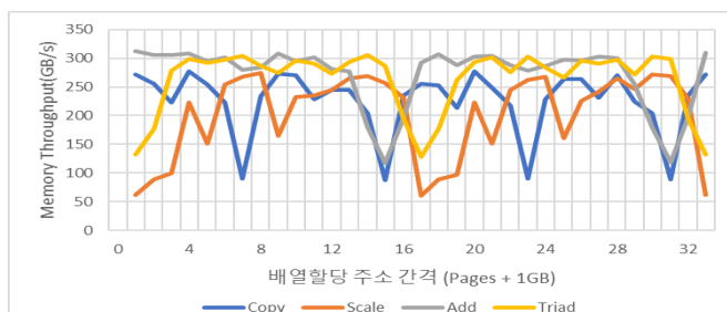
(그림 7) Quadrant 모드에서 배열 간격에 따른 메모리 성능
