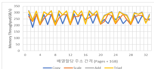
(그림 8) SNC-4 모드에서 배열 간격에 따른 메모리 성능
