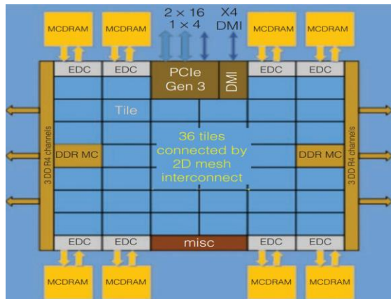
(그림 1) KNL Architecture
