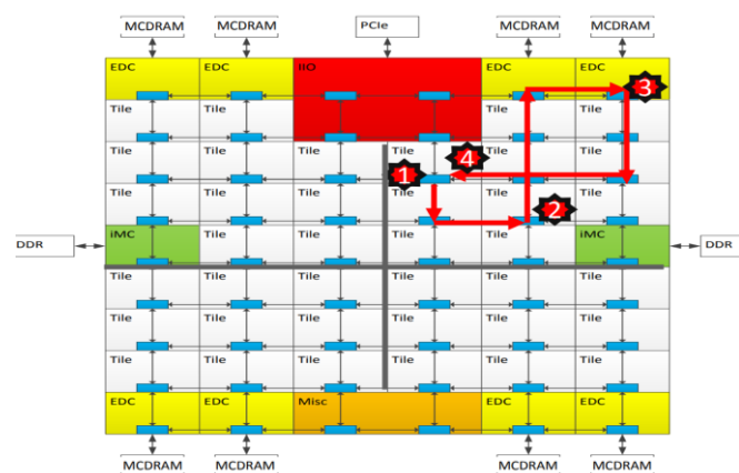
(그림 3) SNC-4 모드에서 메모리 접근 경로
