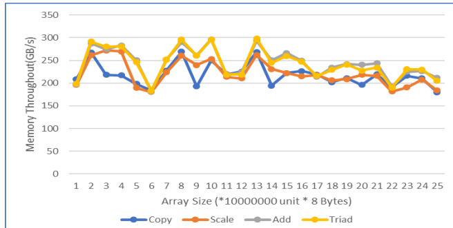
(그림 6) SNC-4 모드에서 배열 크기에 따른 메모리 성능
