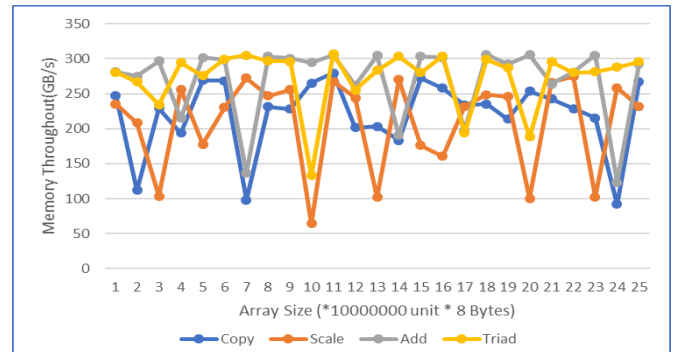
(그림 4) Quadrant 모드에서 배열크기에 따른 메모리 성능
