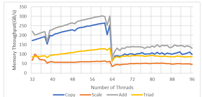
(그림 5) 스레드 개수에 따른 메모리 성능
