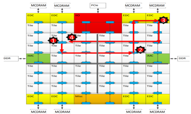
(그림 2) Quadrant 모드에서 메모리 접근 경로
