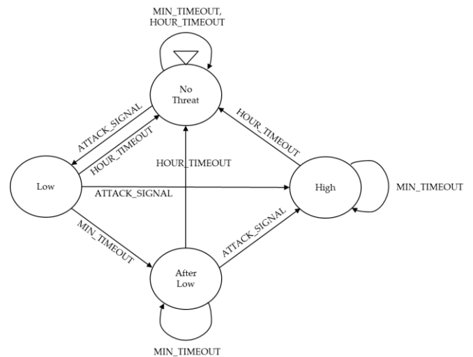
(그림 2) BLACKBOX 에서 사용된 유한 상태 머신[4]
