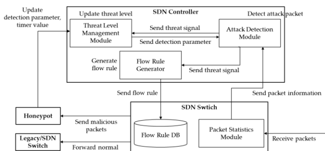
(그림 3) 공격 탐지 및 차단 흐름도
