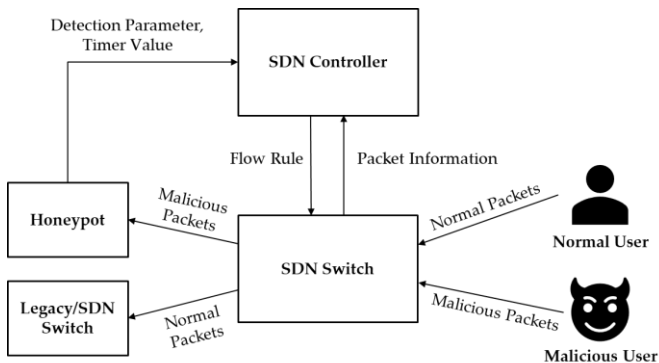
(그림 1) 제안 시스템 구조도.
