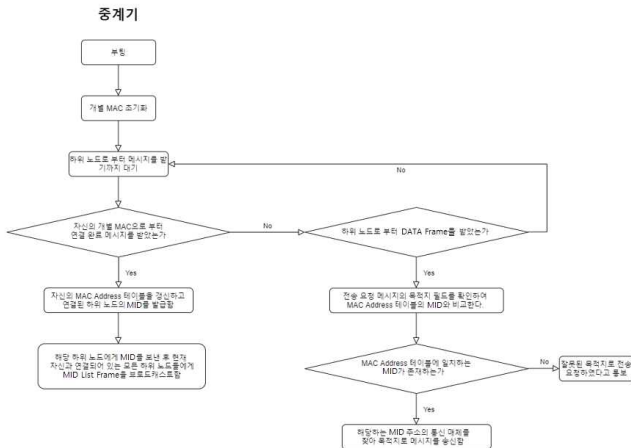
그림 4 중계기 메시지 전송 알고리즘의 흐름도
