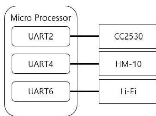
그림5 Mediator 하드웨어 구성도
