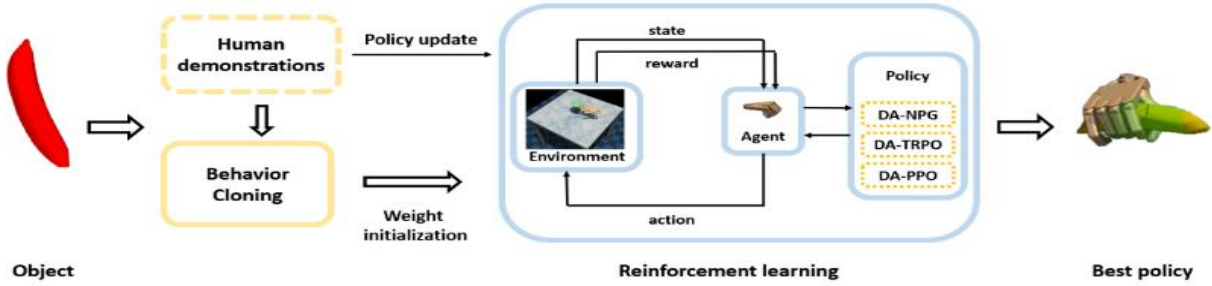
(그림 3) 로봇손 사물 조작(파지 및 재배치) 학습을 위한 전체 강화학습 과정.
