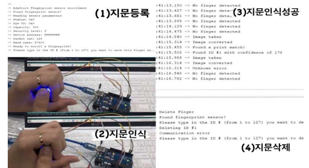
그림. 3 지문 인식 센서 실험 결과.
