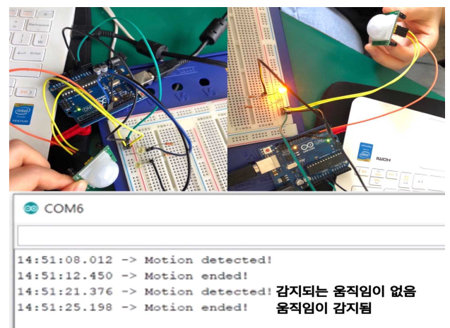
그림. 2 적외선 인체 감지 센서 실험 결과.
