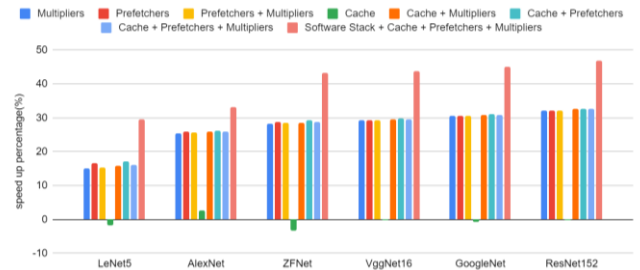
(그림 4) DCNN 워크로드별 각 모듈의 속도 향상
