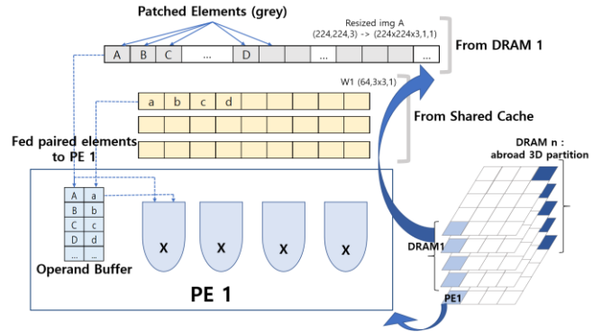
(그림 2) 공유 캐시를 이용한 합성곱 연산 수행 과정
