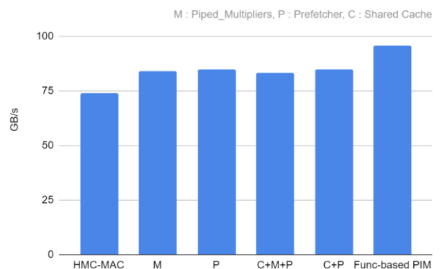
(그림 5) GoogleNet 수행 시, 32 개 PE 에서의 대역폭
