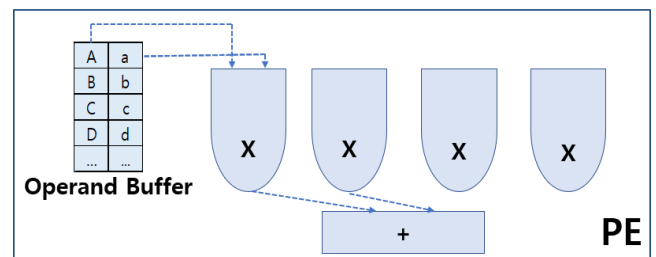
(그림 3) Pipelined Multipliers
