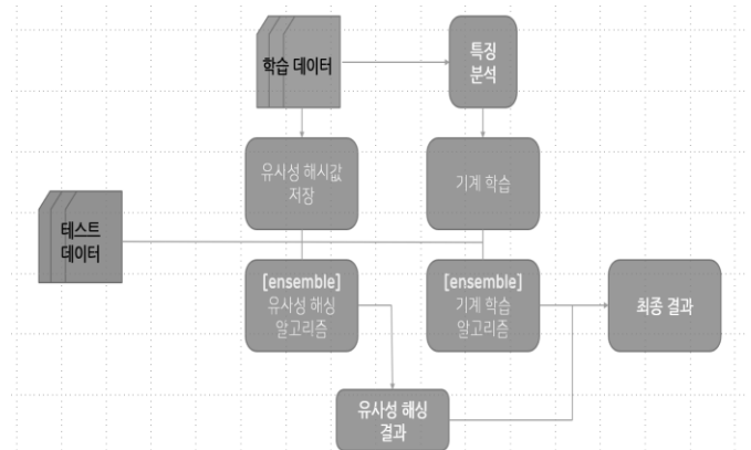
(그림 1) VP-Tree 와 딥러닝을 이용한 탐지 프로세스
