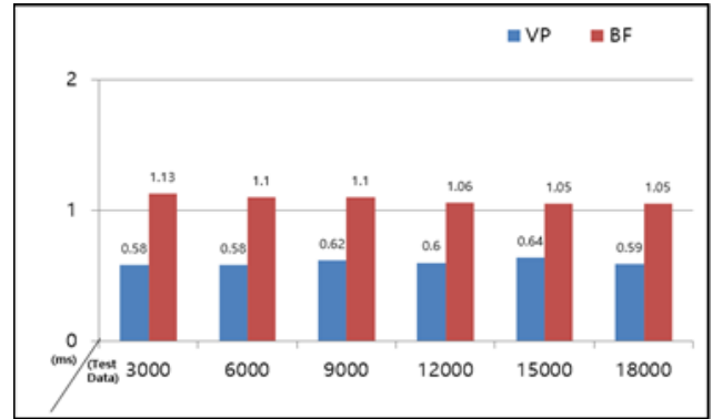
(그림 9-3) 평균 검색시간
