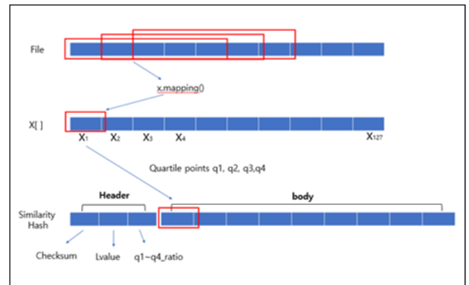
(그림 4) TLSH 사의 유사도해시
