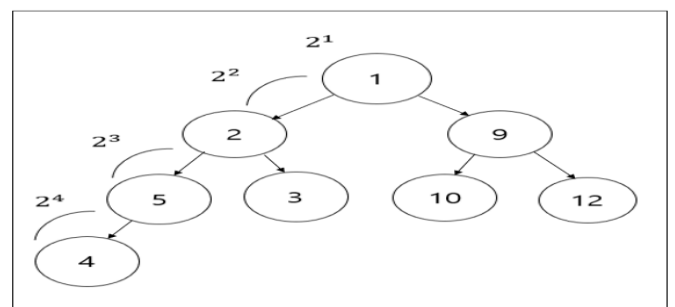
(그림 8-2) VP-Tree
