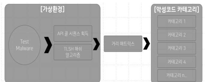
(그림 5) 유사도해시 탐지 모델
