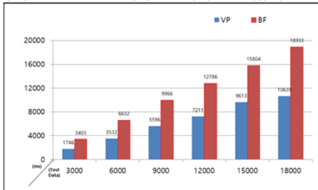
(그림 9-1) 총 검색시간
