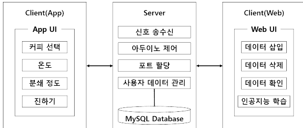
(그림 5) 시스템 구성도.
