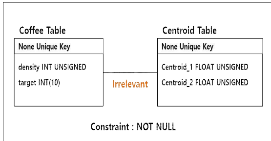
(그림 7) 'ISIADB' 데이터베이스 엔티티관계도.
