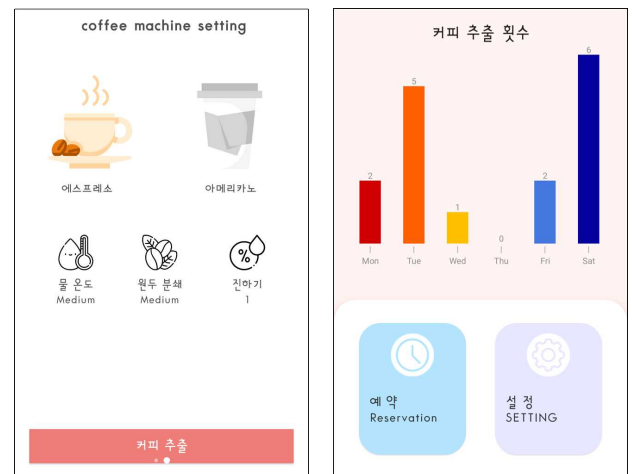
(그림 6) 어플리케이션 UI 메인(왼쪽), 옵션(오른쪽).
