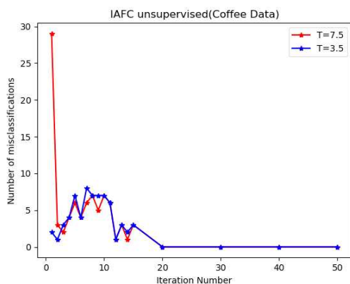
(그림 3) 학습 횟수에 따른 에러의 개수.
