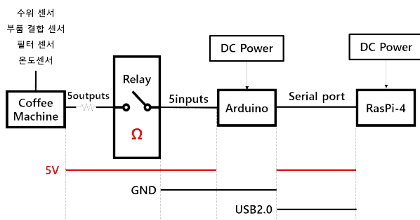
(그림 8) 하드웨어 구성도.
