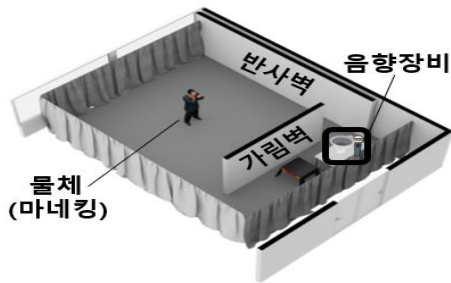
그림 2. 실험실 구조도
