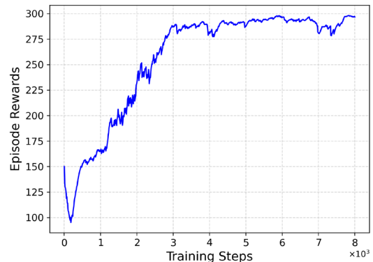
그림 2. 학습 그래프
